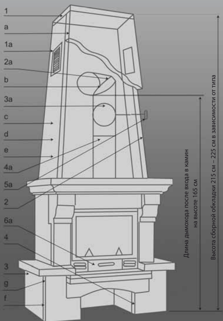
Схемы сборных обкладок
